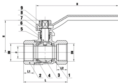
Ausführung IG/IG
