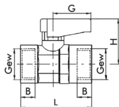
Ausführung IG/IG
